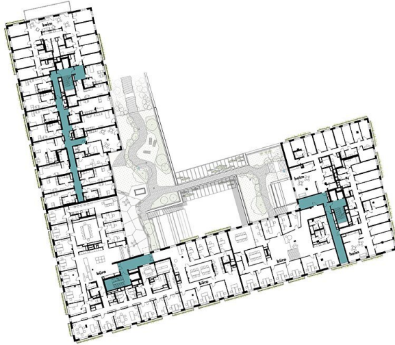
nb1 m 1:400 1.obergeschoß 09.04.2024
