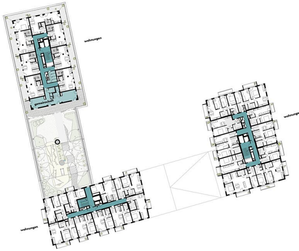
5.obergeschoß nb1 m 1:400 09.04.2024
