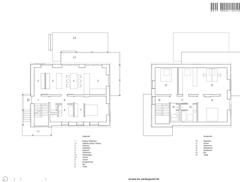
Grundrisse EG, OG
