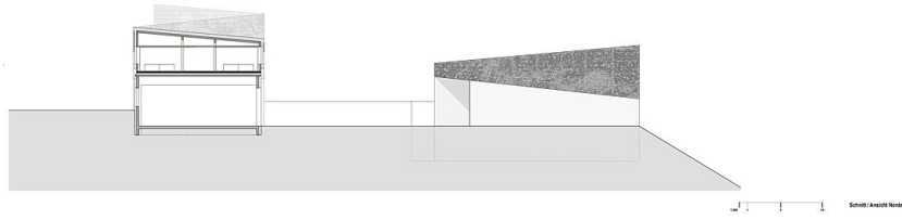
Schnitt, Ansicht Nord
