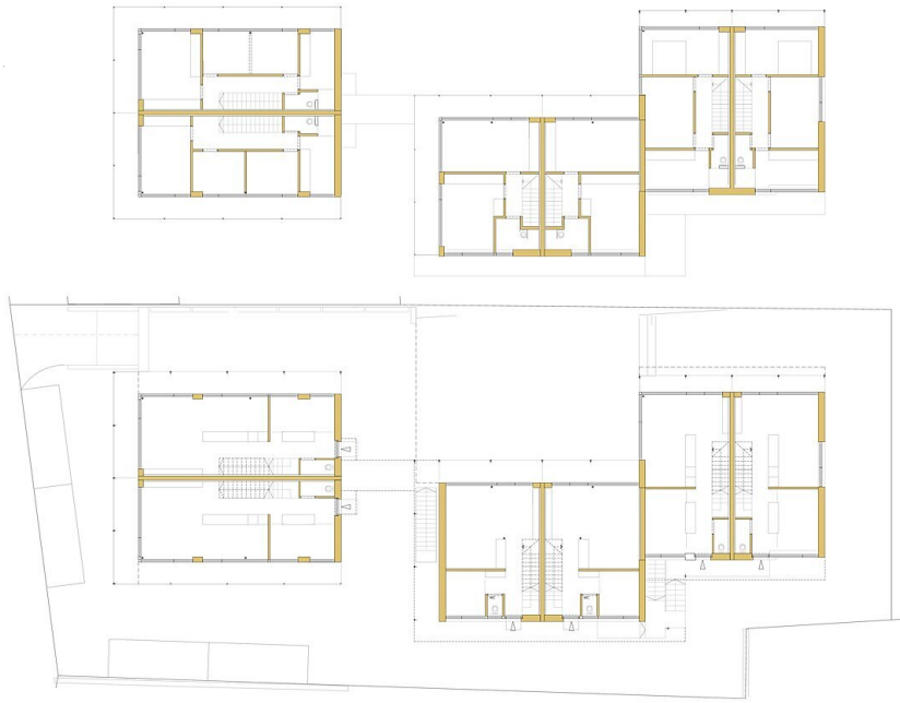
Grundrisse
