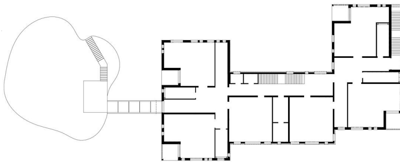
Grundriss OG
