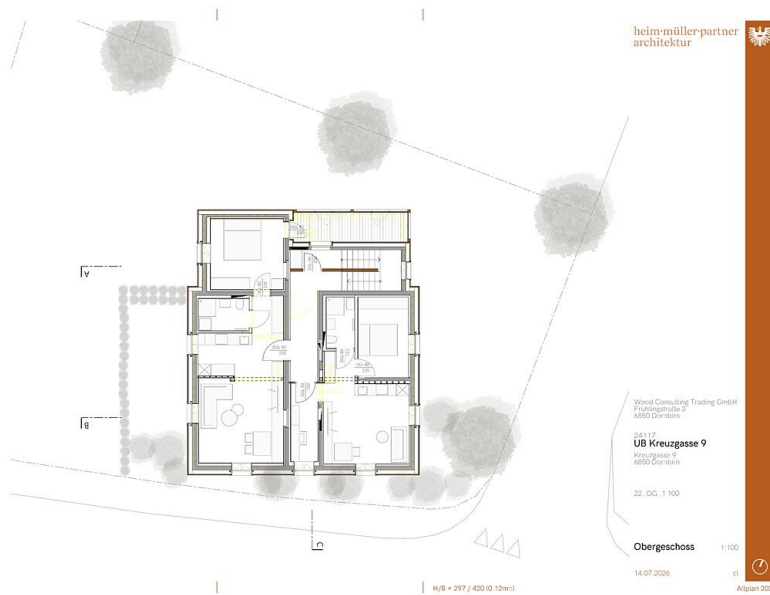
Grundriss OG
