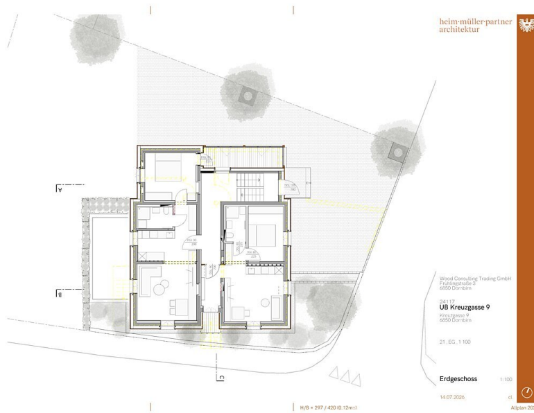
Grundriss EG
