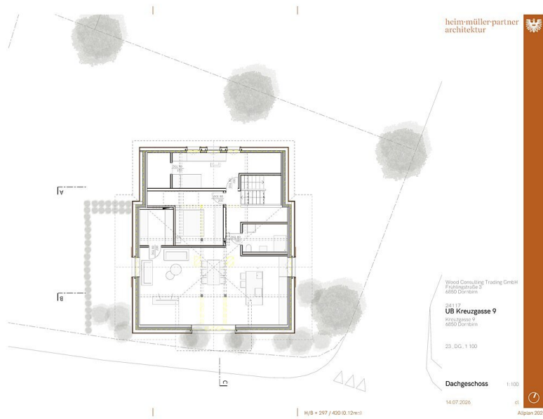
Grundriss DG
