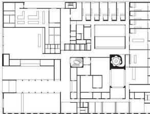
Alters- und Pflegezentrum Zehntfeld Widnau - Ebene 2
