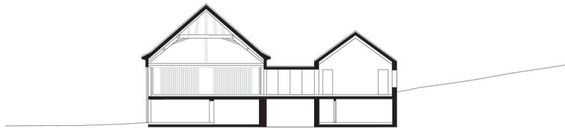
Querschnitt 1
