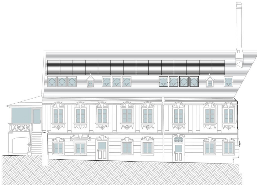
Ansicht West
