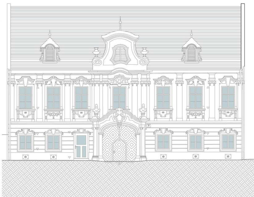
Ansicht Süd
