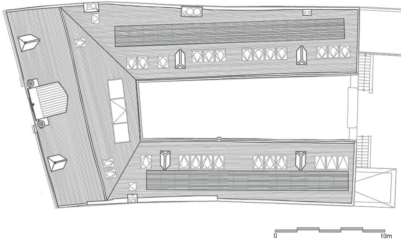
Dachaufsicht
