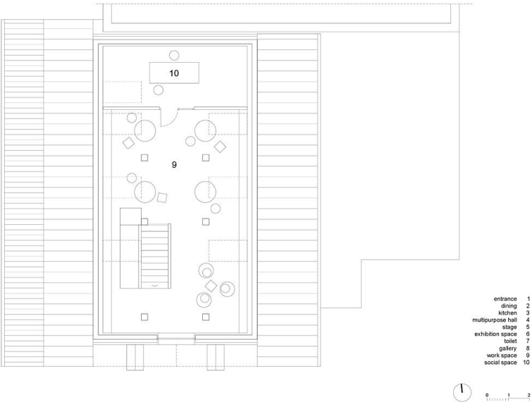
Grundriss DG
