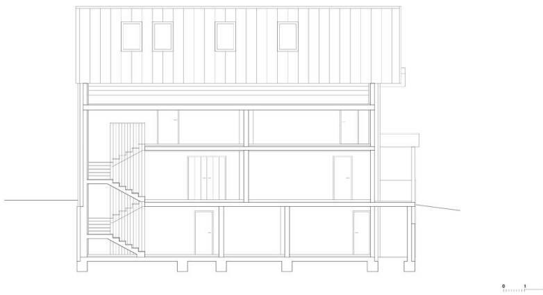
Schnitt BB
