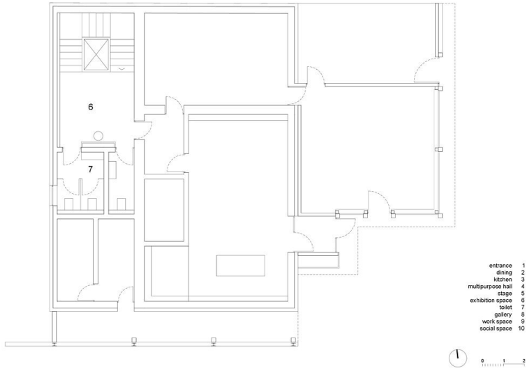
Grundriss UG
