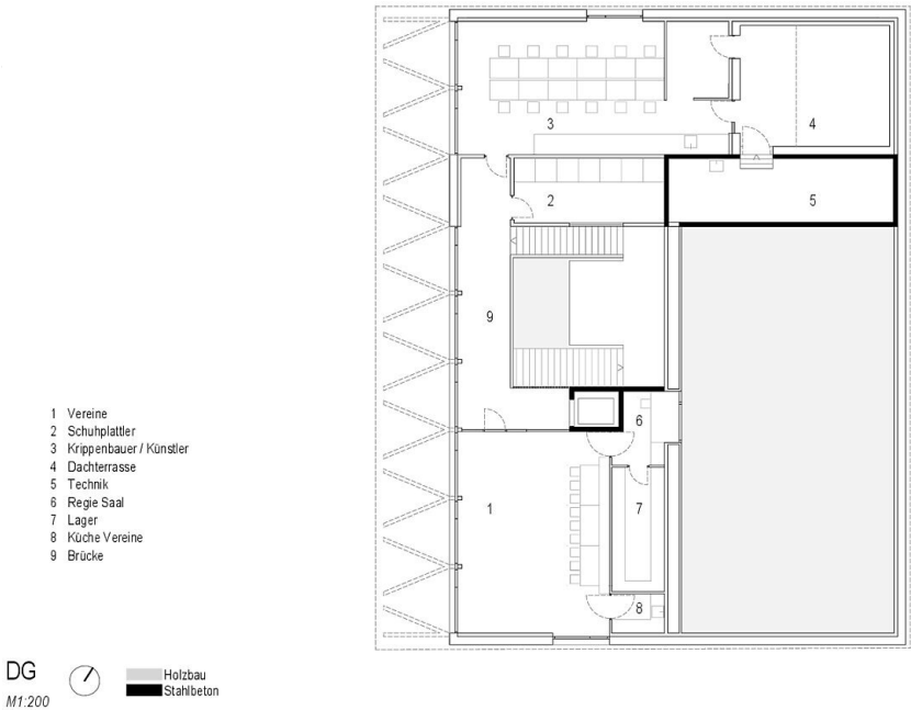
Grundriss DG
