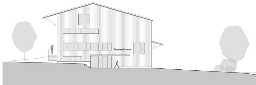
Ansicht SÜD M1:200
