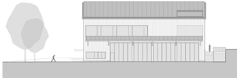
Ansicht OST M1:200
