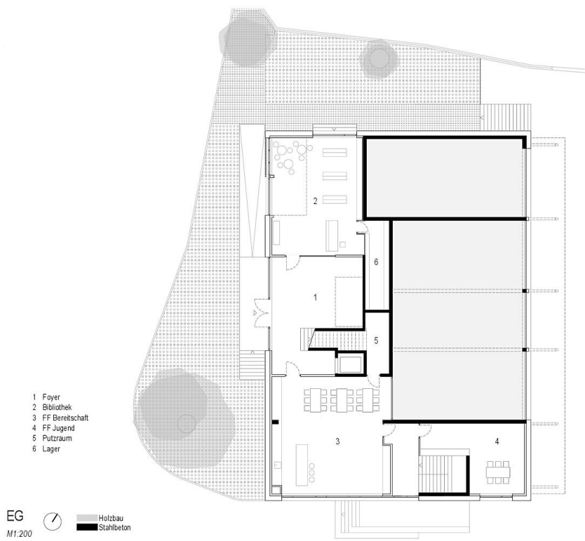
Grundriss EG
