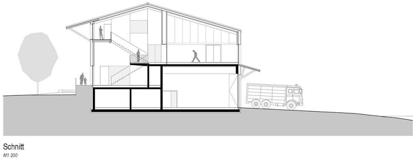
Schnitt
