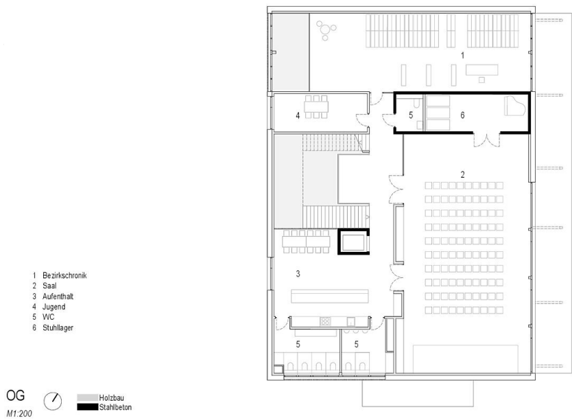
Grundriss OG
