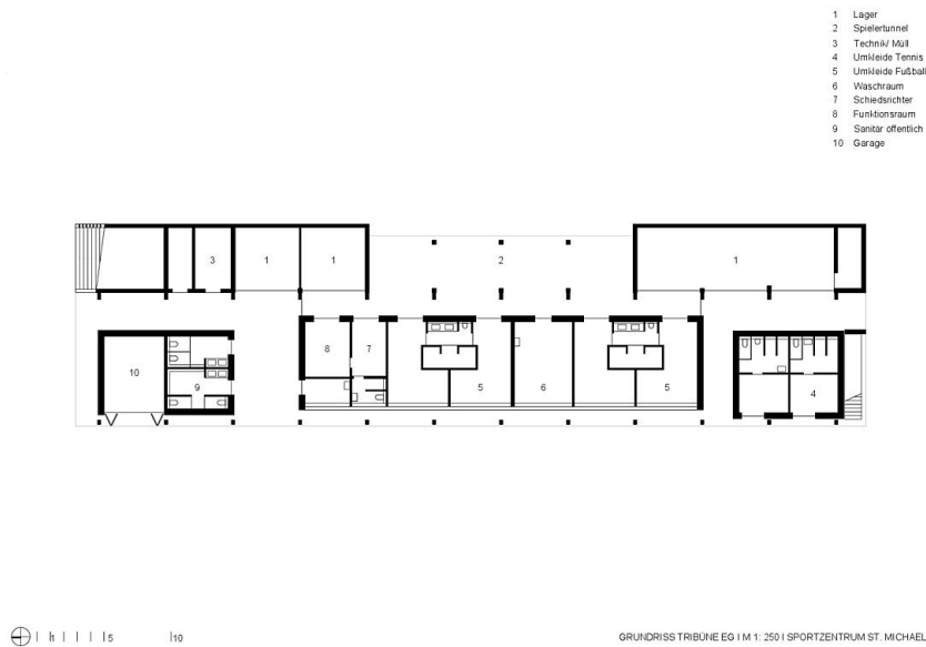
Grundriss EG
