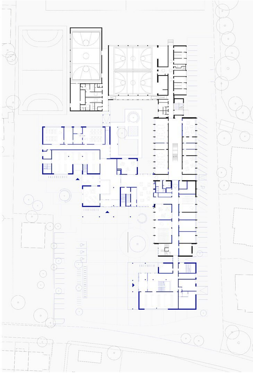
Grundriss EG
