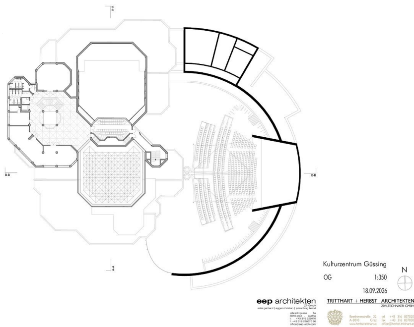
Grundriss OG
