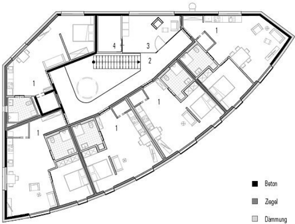
Obergeschoss
