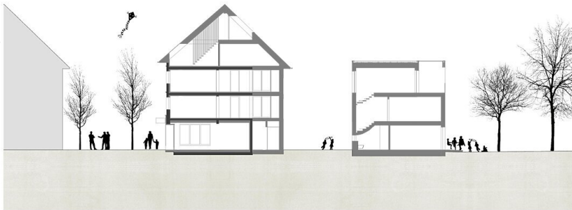
Längsschnitt Marktstraße 52a
