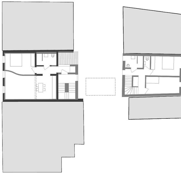
Grundriss Obergeschoss 1
