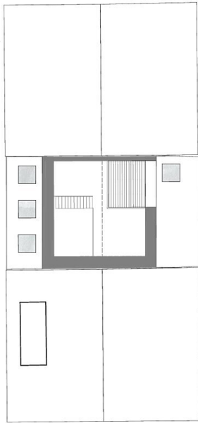
Grundriss Dachgeschoss
