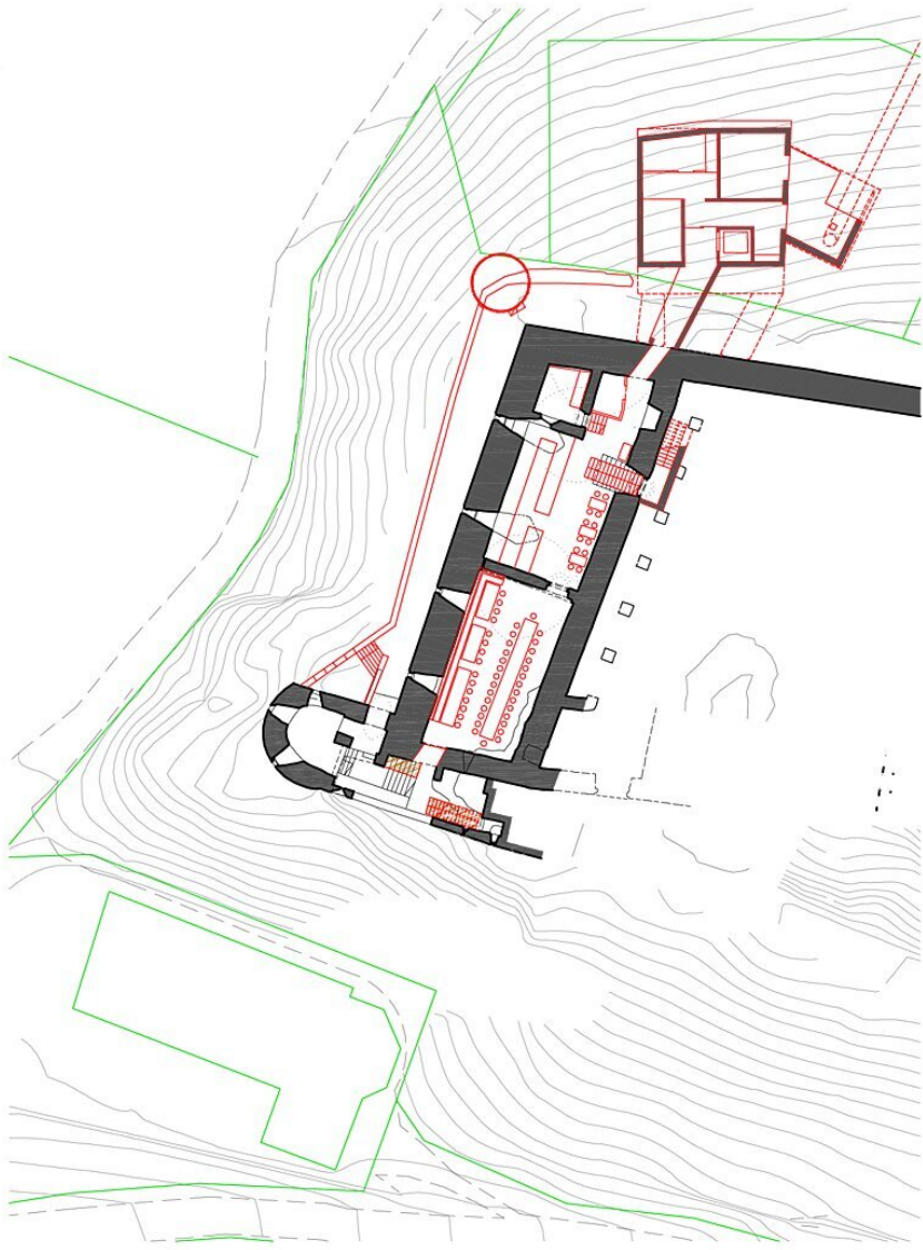
BURG HEINFELS - UNTERGESCHOSS 0 2 10 20 N
