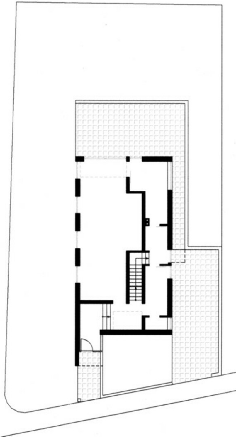
Grundriss OG
