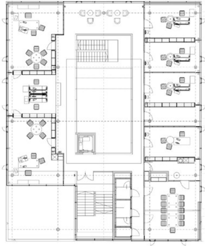
Grundriss OG1
