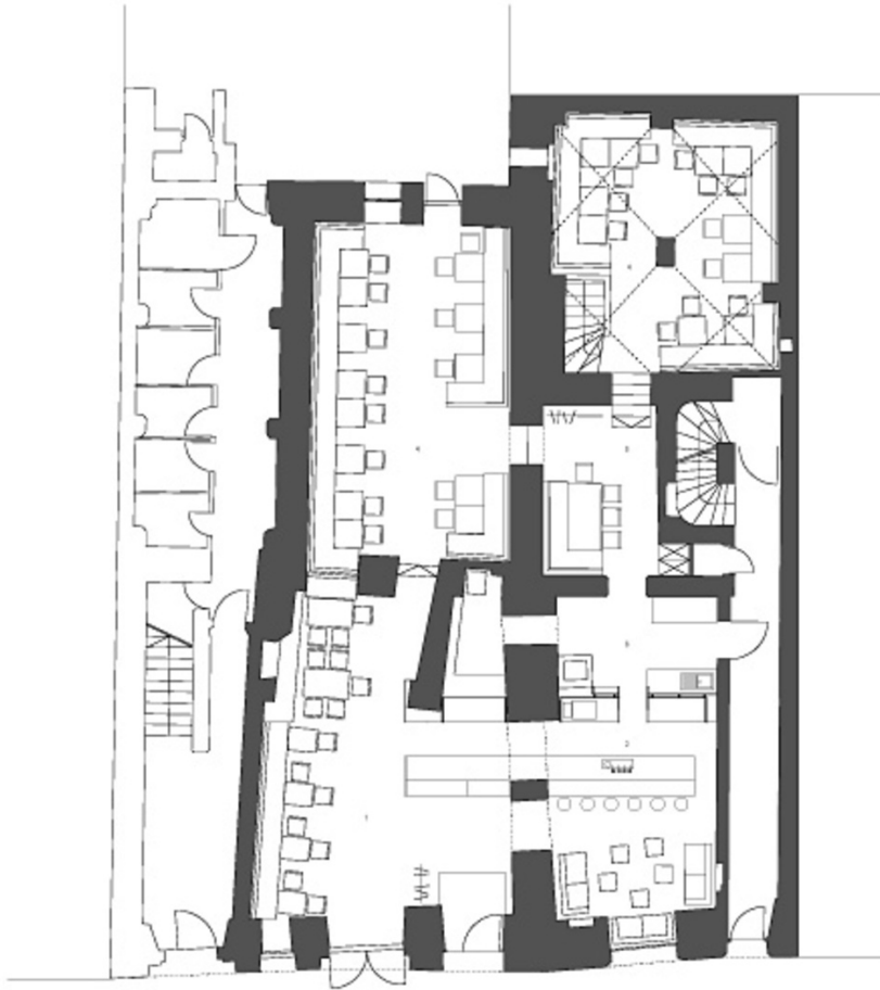
Grundriss
