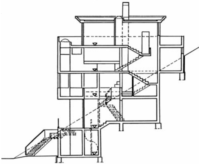
Schnitt
