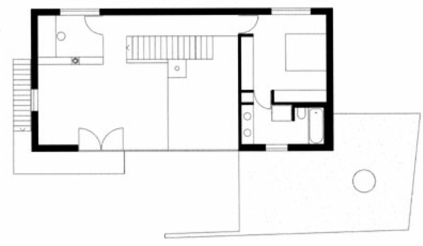
Grundriss OG
